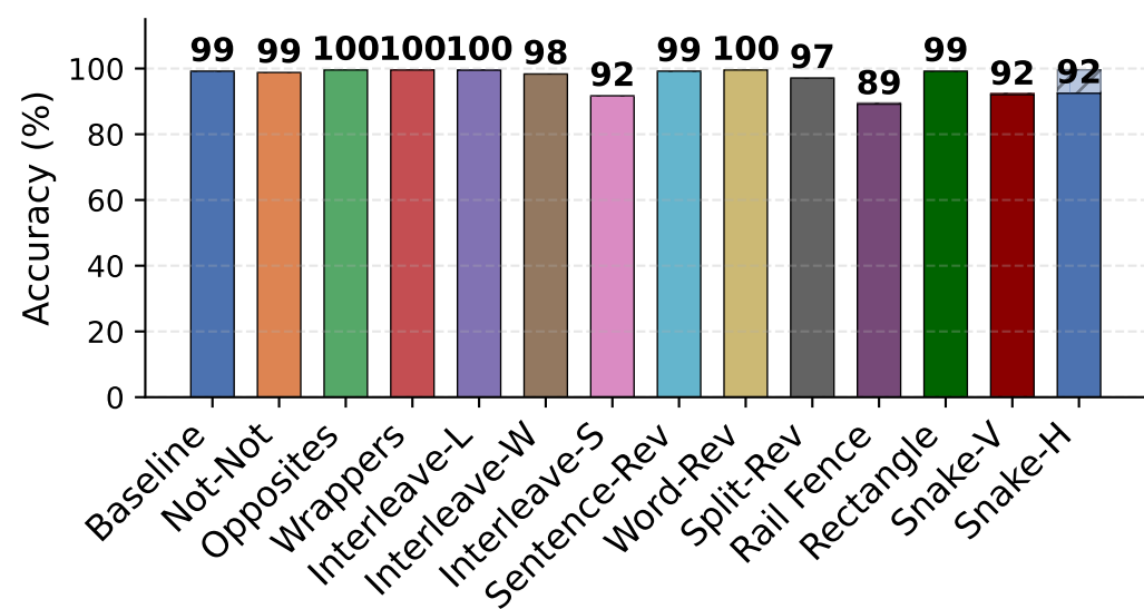
Claude Opus 4.6
