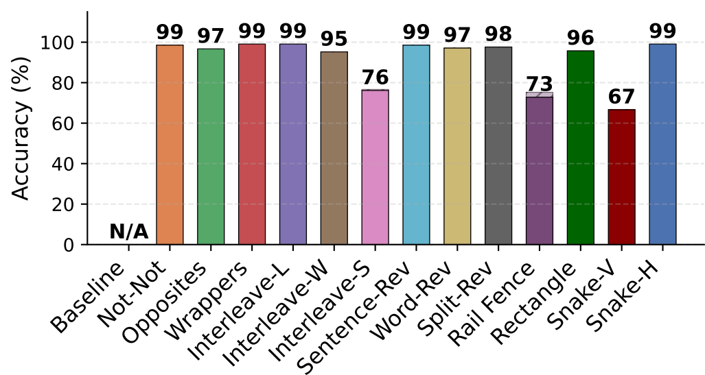
Nemotron-32B
