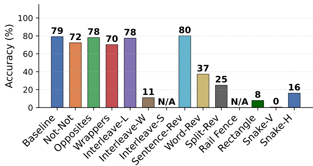
Qwen3-30B-A3B
